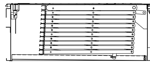
梯子納まり図
