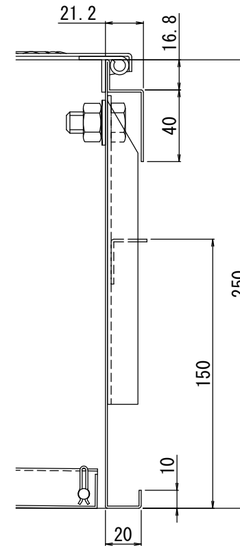
吊元詳細(1:3)
