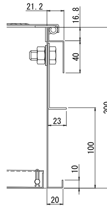
吊元詳細(1:3)
